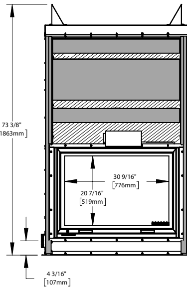
VUE FRONTALE
