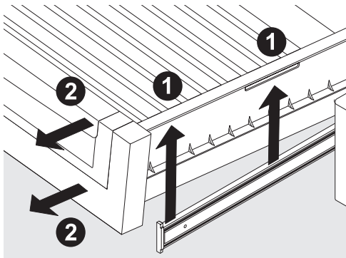
Figure 40 Retrait du tiroir
