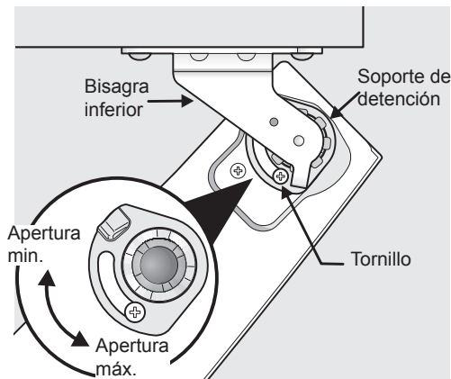
Tope ajustable para la puerta Figura 15
