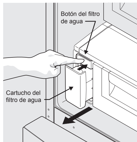
Figura 49 Oprima el botón del filtro de agua
