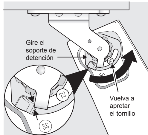
Vuelva a apretar el tornillo Figura 17
