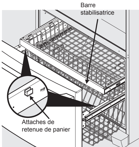
Les deux paniers du congélateur
