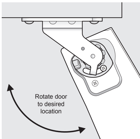
Adjusting door
