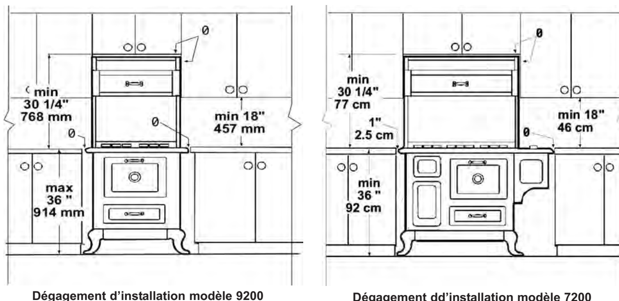
Figure 2 Dégagements d'installation
