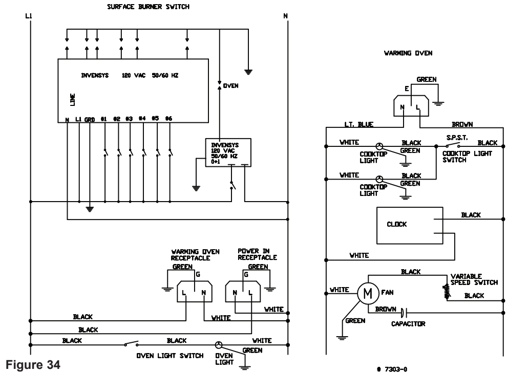
7200 WIRING DIAGRAM - N.A.
